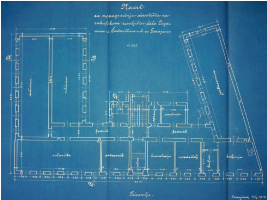
Sl. 1. Nacrt prizemlja zgrade sirotišta (ABiH, ZVS, 1912, kut. 762, sign. 248-182)
