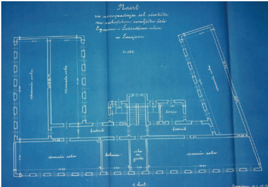
Sl. 2. Nacrt prvog sprata zgrade sirotišta (ABiH, ZVS, 1912, kut. 762, sign. 248-182)
